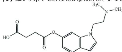
(5) Izo-N,N dimetiltriptamin-6-sukcinata
