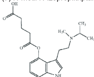
(7) N-metil N-izopropiltriptamin-4-glutarata
