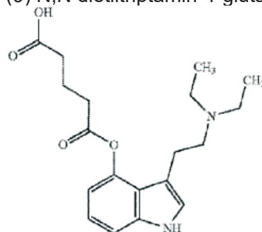
(9) N,N dietiltriptamin-4-glutarata
