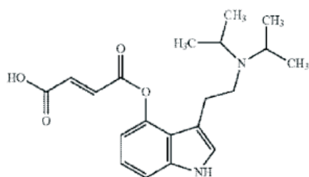
(4) Psilocin-4-metil-5-sukcinata
