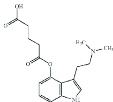
(9) N,N dietiltriptamin-4-glutarata
