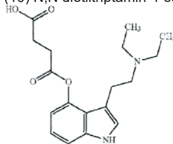
(10) N,N dietiltriptamin-4-sukcinata
