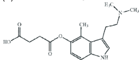
(4) Psilocin-4-metil-5-sukcinata
